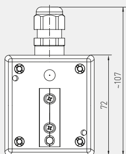
Габаритный чертеж
