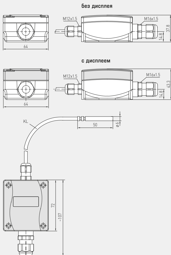
Габаритный чертеж
