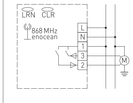
Схема подключения
