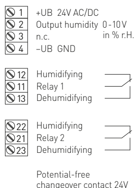
Схема соединения
