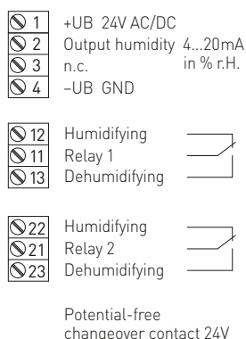
Схема соединения
