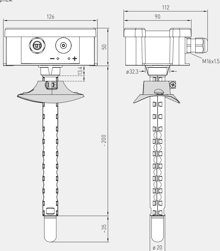
Габаритный чертеж
