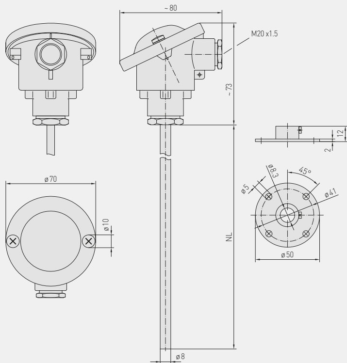
Габаритный чертеж
