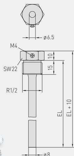
Габаритный чертеж
