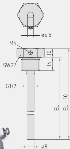
Габаритный чертеж
